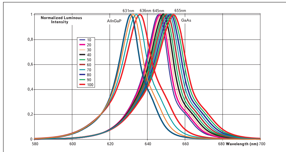
Рис. 2. Относительные спектральные характеристики излучения светодиодов красного цвета на кристаллах различных типов. В верхней части графика указан разброс максимальной длины волны L_{max} в зависимости от прямого тока (приведен на вставке в мА)
