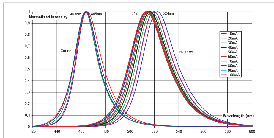
Рис. 4. Относительные спектральные характеристики излучения светодиодов зеленого и синего цветов на кристаллах с гетероструктурами InGaN/AlGaIn/GaN. В верхней части графика указан разброс максимальной длины волны \lambda_{max} в зависимости от прямого тока (приведен на вставке)
