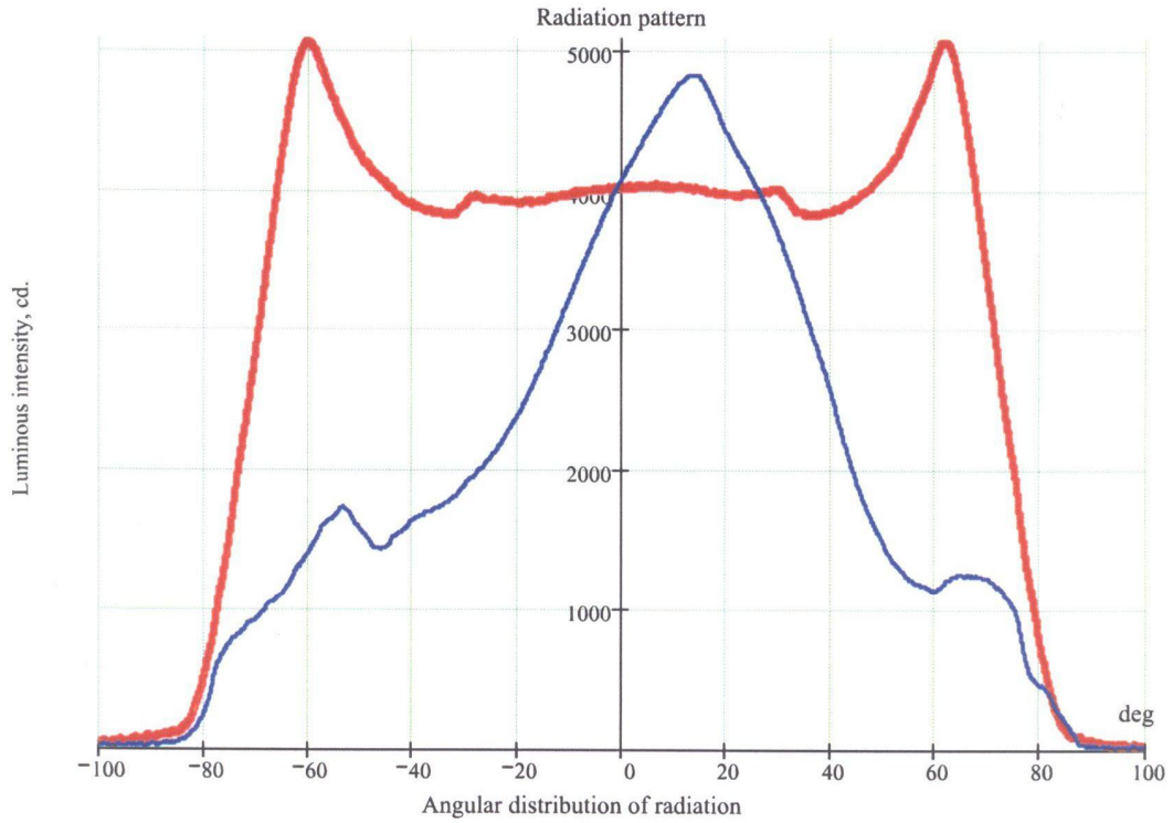
Фотометрические характеристики.
